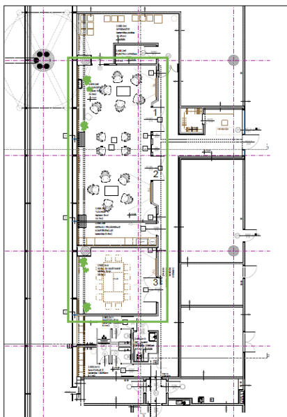
Tlocrt 3b VIP salona 3
