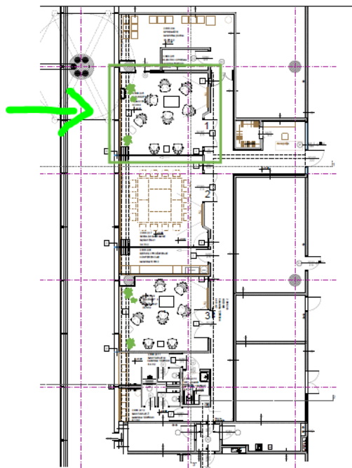
Tlocrt 1a VIP salona 1
